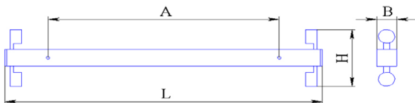
Рис. 1 - ОБН01-2х30-111 Фотон
