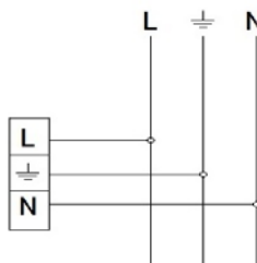
Рис.2 – Схема подключения к сети
