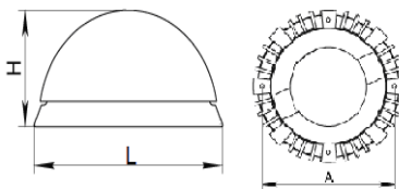
Рис. 1. - Общий вид светильника Vega LED
