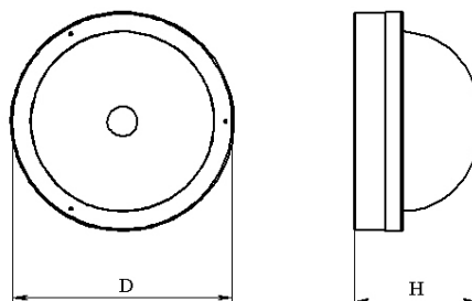
Рис. 1. Общий вид светильника НПП03-100 Стандарт
