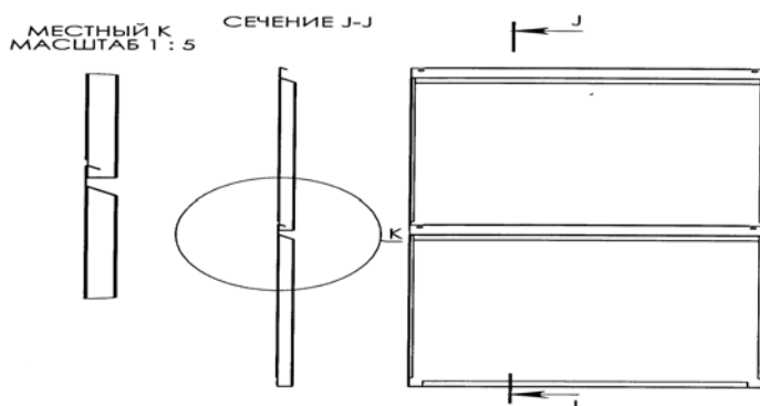
Рис.1 Монтаж кассет.
